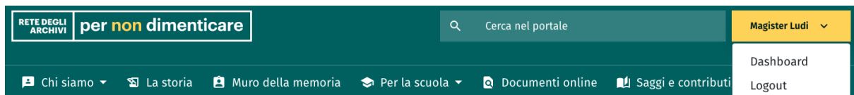
Figura 3 - Menu contestuale
